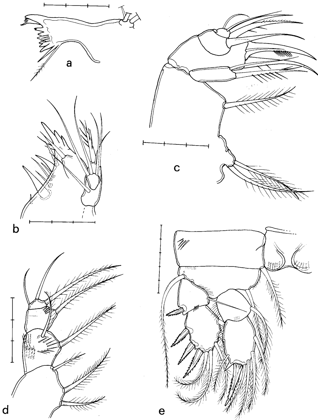
Fig. 2. Diacyclops cohabitatus female : a) mandible ; b) maxillule ; c) maxilla ; d) maxilliped ; e) P1. Scale bars : 50 \mu m (e), 30 \mu m (a,b,c,d).
